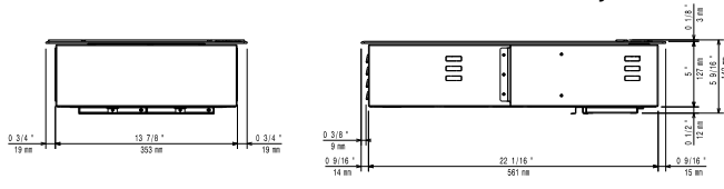
Zij aanzicht
